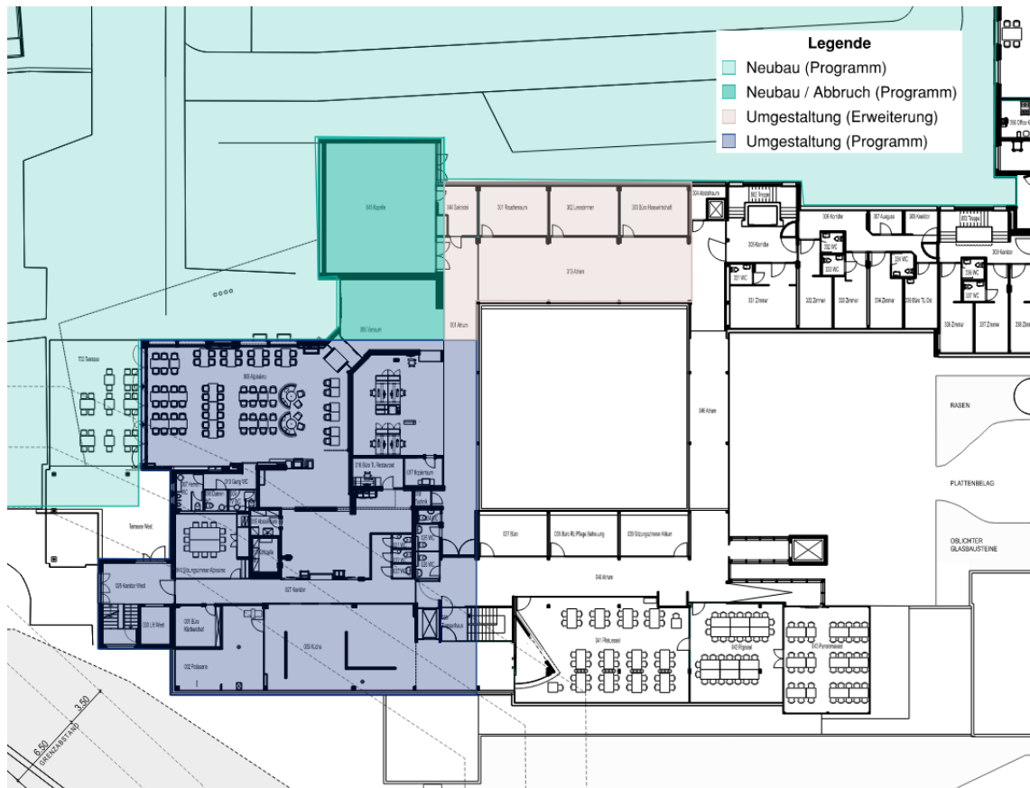
Abbildung 5: Planungsperimeter erweitert (nicht massstäblich)
