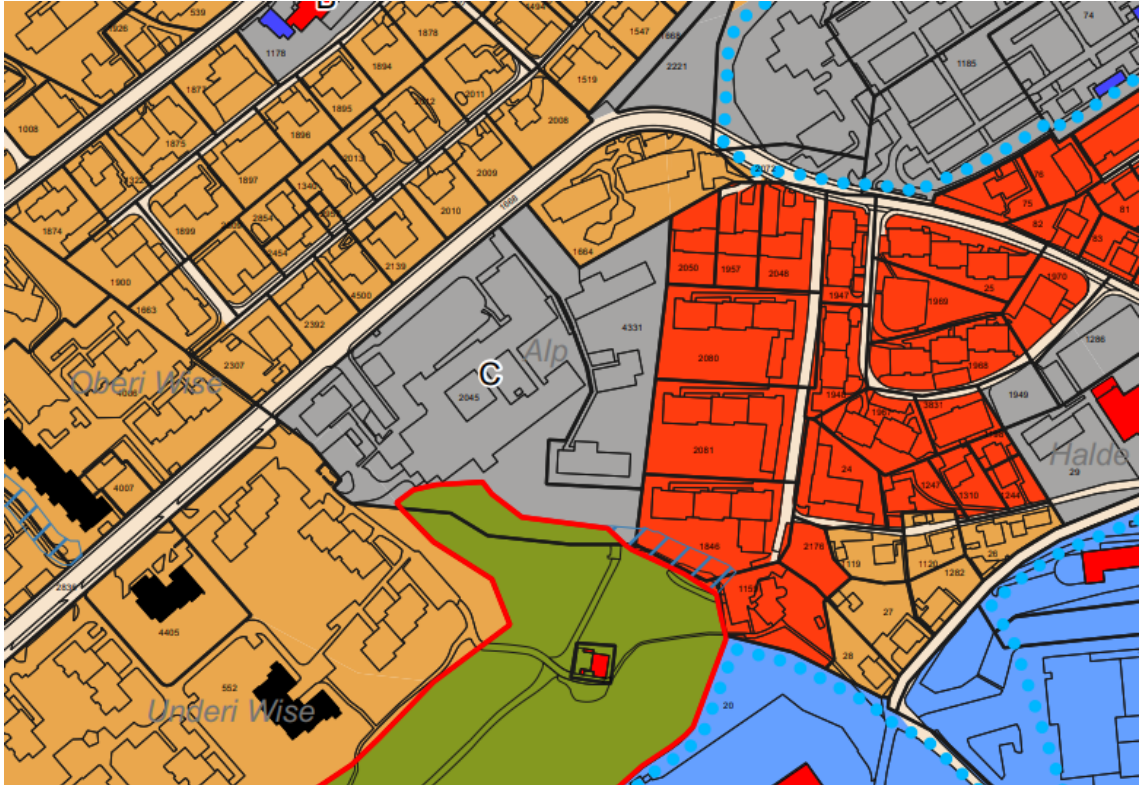
Abbildung 3: Ausschnitt revidierter Zonenplan (nicht massstäblich)
